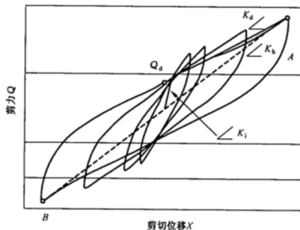
图 E.1 高阻尼橡胶支座的剪力-剪切位移滞回曲线
