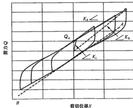
图 E.3 铅芯橡胶支座的剪力-剪切位移滞回曲线
